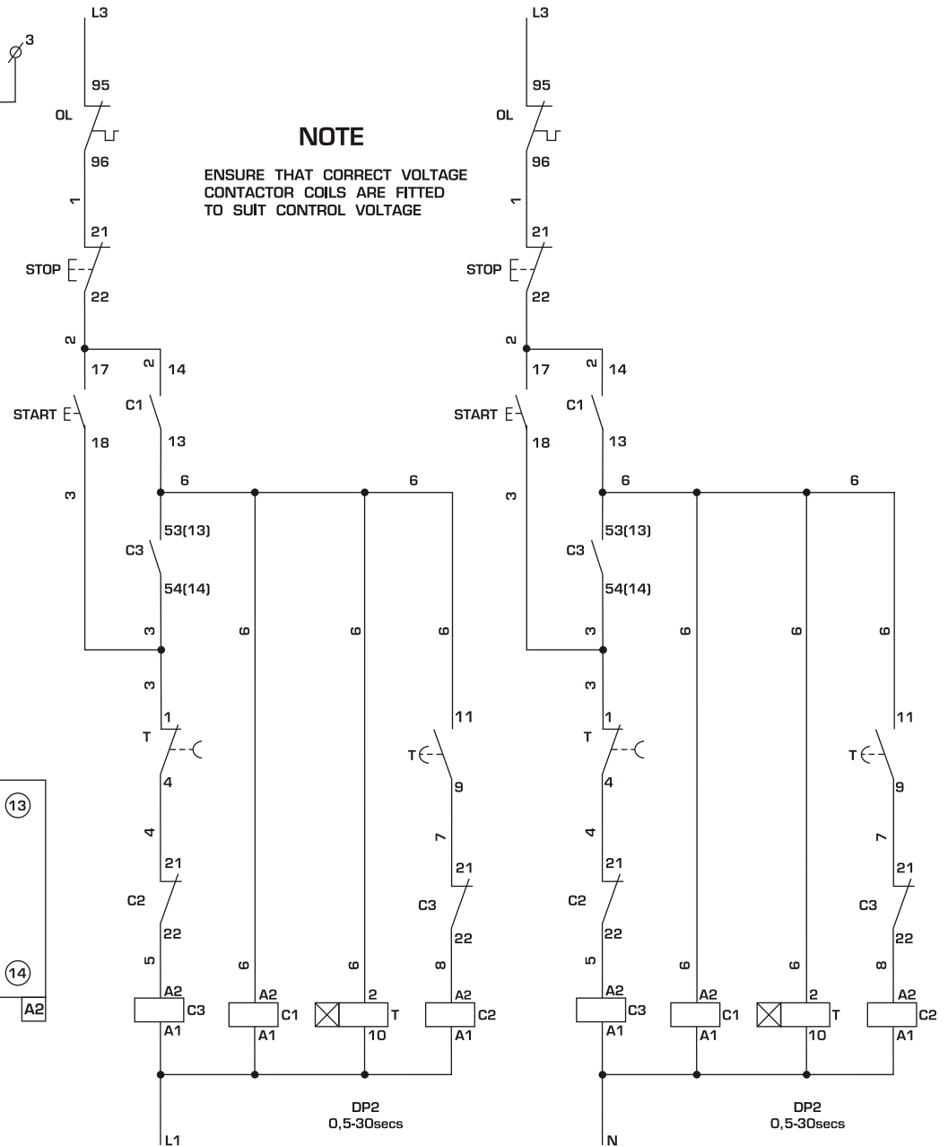
FOR 400 OR 525 VOLT CONTROL
